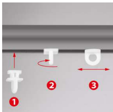
Пл. скользящая петля TWIST вставная-поворотная для крючка и мет. зажима Цвет белый Nr.100
